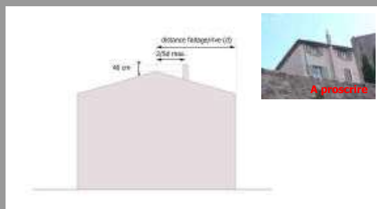
Implantation des conduits de cheminées
