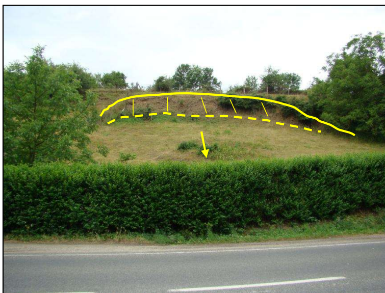
Figure 16 : Talus présentant des instabilités (ondulations à gauche et niche d'arrachement à droite), en face du parking du boulodrome [Source : IMS RN ]
