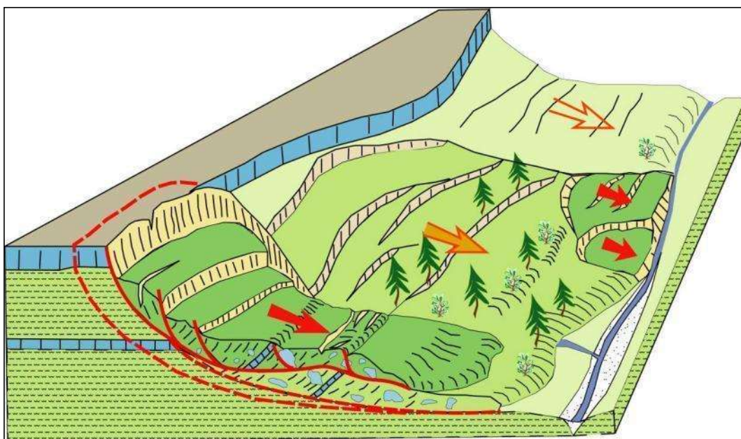
Figure 13 : Schéma conceptuel du phénomène glissement de terrain [Source : IMS RN ]
