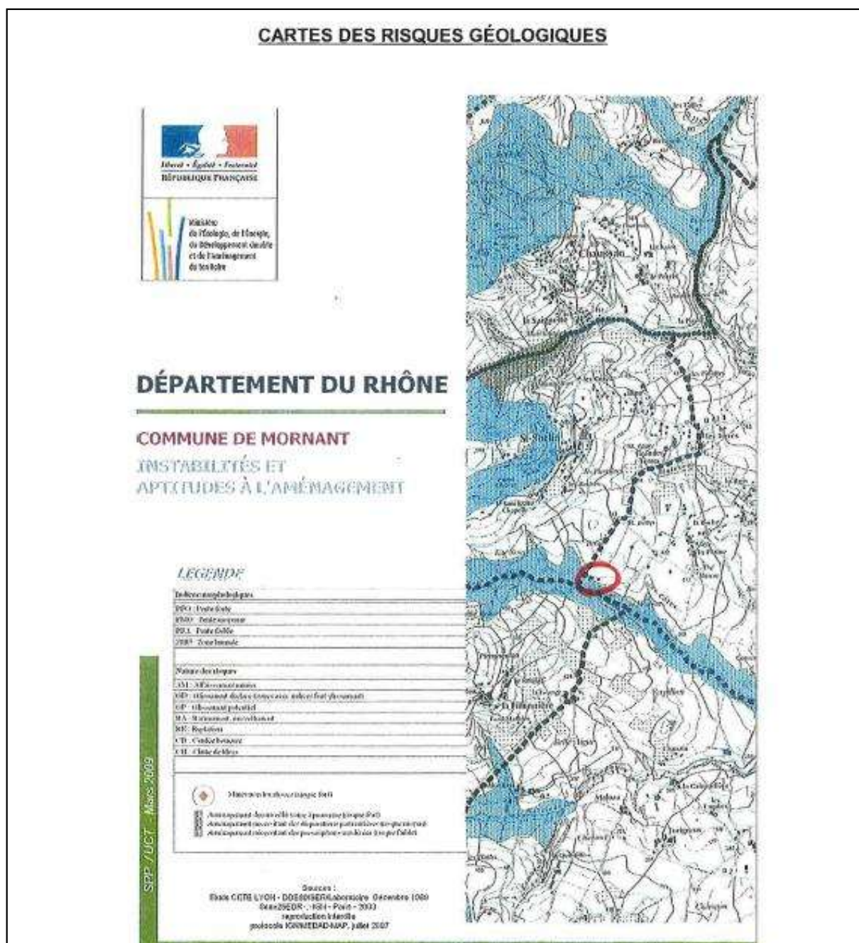
Figure 8 : Cartographie des zones à risques identifiées par le CETE en 1989 [Source : Etude HYDROGEOTECHNIQUE – Octobre 2008]
