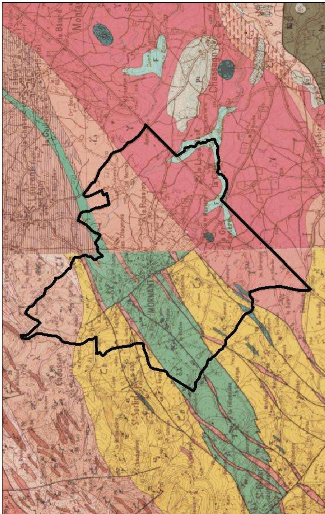
Figure 5 : Carte géologique de la commune de MORNANT [Source : BRGM]
