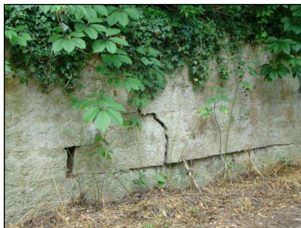
Figure 19 : Mur de soutènement très fissuré (du fait de la poussée des terrains) en bas du chemin des Bines
